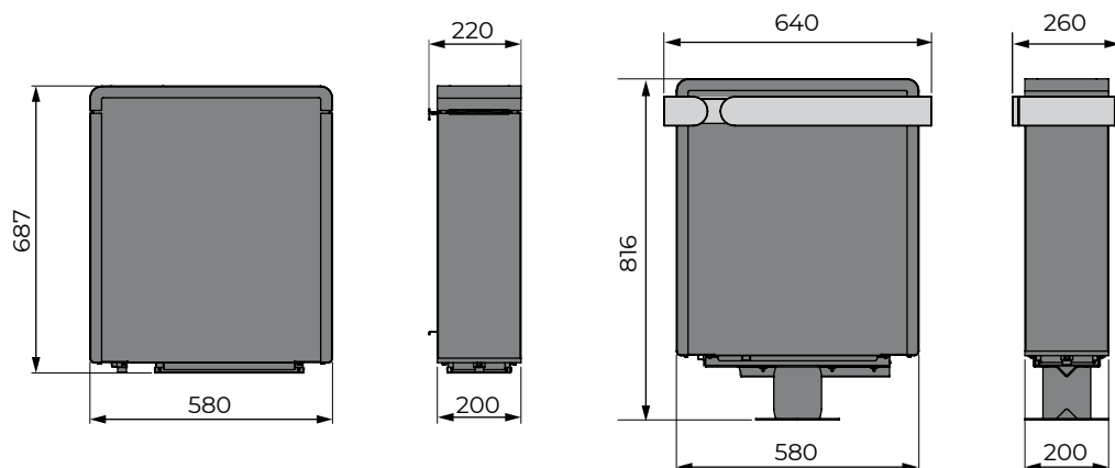
Dimensions of Concept R Mini Combi sauna heaters (CP-RMC-35 / CP-RMC-45 / CR-RMC-60 / CP-RMC-75)
